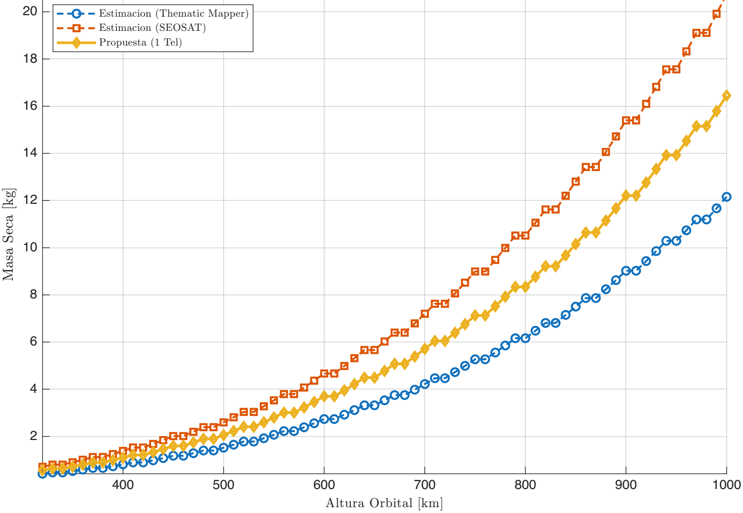
Comparativa de Masa Seca vs. Altura Config: 3 Sat, 1 Tel, Det 1, Refractivo
